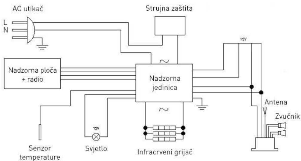
HEMA STRUJNOG KRUGA
