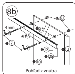
Imbusovým kľúčom 4mm utiahneme šróby 6.3 a nasunieme krytky č.7
