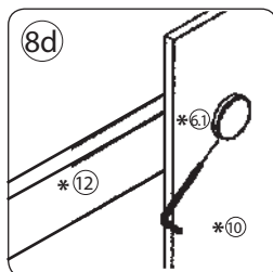
Do otvoru dielu 6.1 z bočnej strany vsunieme imbusový kľúč (4mm)
