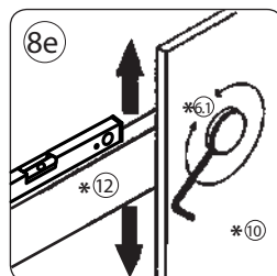
Pootočením imbusového kľúča do strán, štelujeme vodiaci profil č.12 do roviny.
